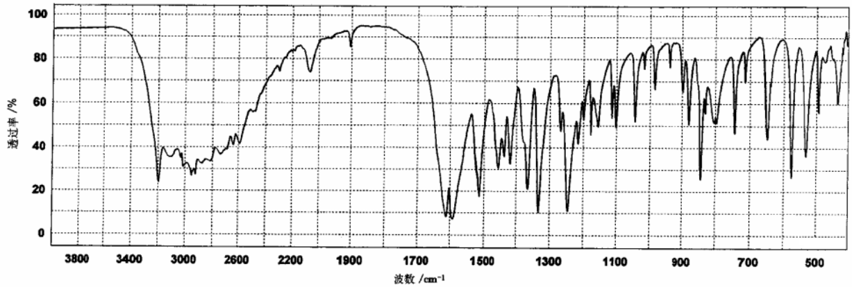
图A.1 天(门)冬氨酸标准品红外吸收光谱图
