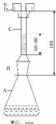
图1 仪器装置
