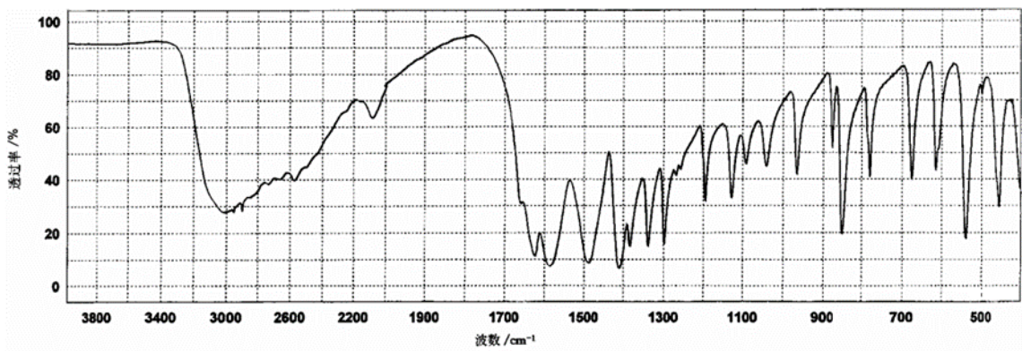
图A.1 胱氨酸标准品红外吸收光谱图
